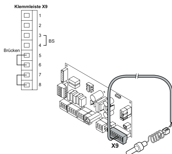
Bild 23 Schaltplan Warmwasserheizschlangensensor bzw. -thermostat
