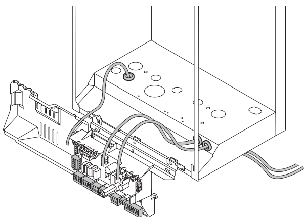
Bild 18 Anschluss externer Steuerungen LT.AL.W7H.000.024
