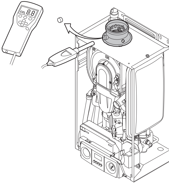
Bild 49 Kontrolle der Verbrennung 111572.LT.DE.W7H.029
