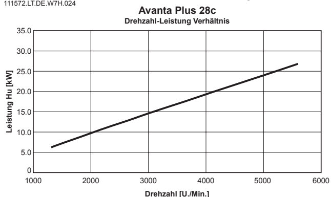
Bild 42 Gebläsedrehzahl/Kesselleistung AvantaPlus 28c 111581.LT.DE.W7H.002
