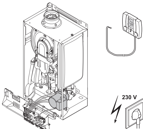
Bild 33 Einschalten und Steuerung bei Wärmeanforderung 111572.LT.DE.W7H.019
