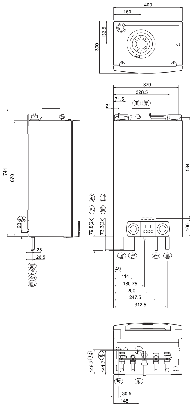
Bild 05 Abmessungen und Anschlüsse für Remeha AvantaPlus Combi
