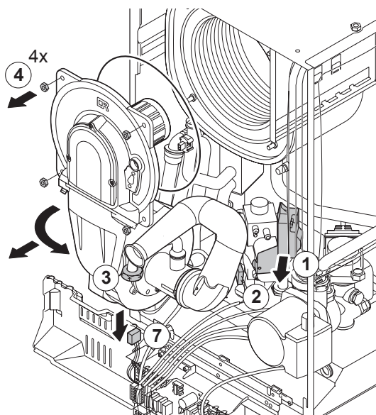
Bild 52 Demontage der Frontplatte des Wärmetauschers
