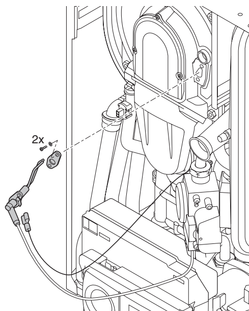
Bild 51 Wartung der Elektrode LT.AL.W7H.000.059
