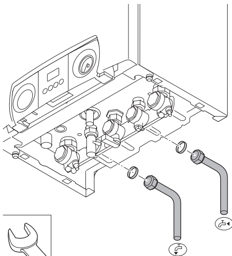
Bild 08 Anschluss Warmwasserleitungen LT.AL.W7H.000.015
