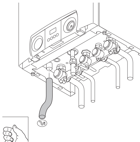
Bild 11 Anschluss Kondensatableitung LT.AL.W7H.000.018
