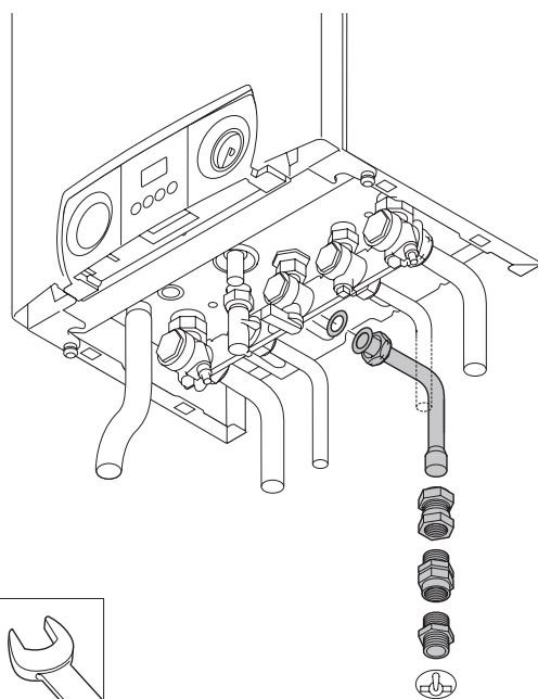
Bild 12 Anschluss Gasleitung 111572.LT.DE.W7H.003
