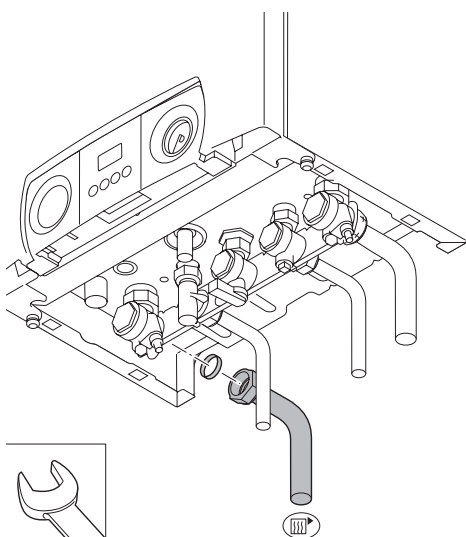
Bild 10 Anschluss Heizungsvorlauf LT.AL.W7H.000.017
