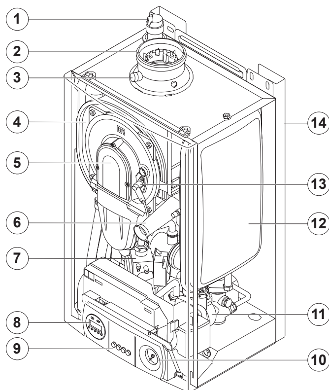
Bild 59 Bauteile Remeha AvantaPlus Combi LT.AL.W7H.000.202
