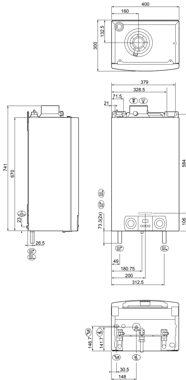
Bild 04 Abmessungen und Anschlüsse für Remeha AvantaPlus Solo
