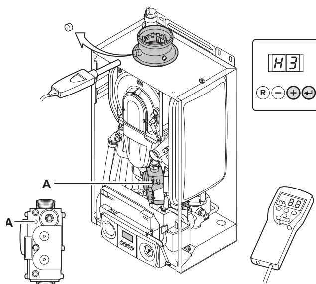
Bild 34 Prüfung der Gas-/Luftverhältnissteuerung – bei Volllast – Gas-/Luftverhältnis Einstellung A am Gasblock 111572.LT.DE.W7H.020
