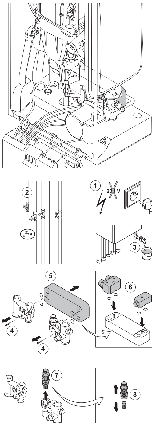
Bild 55 Reinigen des Plattenwärmetauschers und des Rückschlagventils mit Filter
