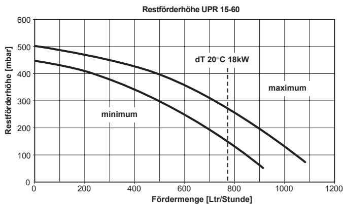
Bild 07 Grafik Pumpe UPR 15-60 für die ZH-Installation mit AvantaPlus 24s und 28c 111572.LT.DE.W7H.002
