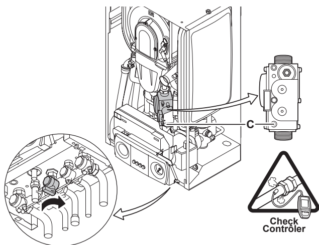
Bild 31 Messpunkt c am Gasblock LT.AL.V7H.000.039
