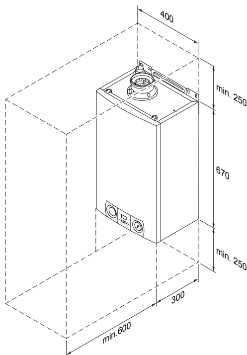
Bild 03 Platzbedarf und Abstände
