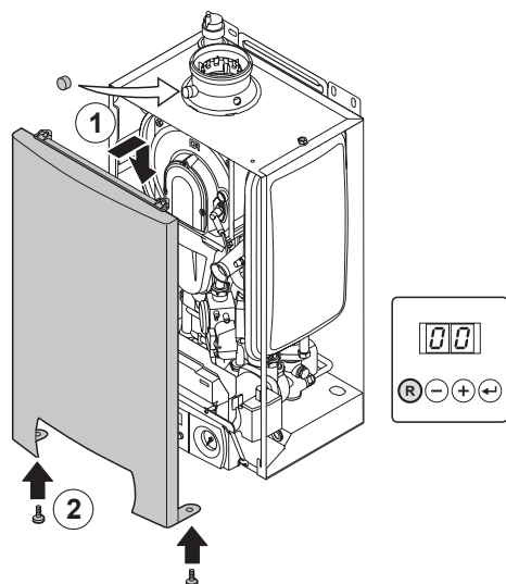
Bild 36 Inbetriebnahme des Kessels 111572.LT.DE.W7H.022
