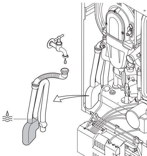
Bild 47 Kontrolle des Siphons LT.AL.W7H.000.233
