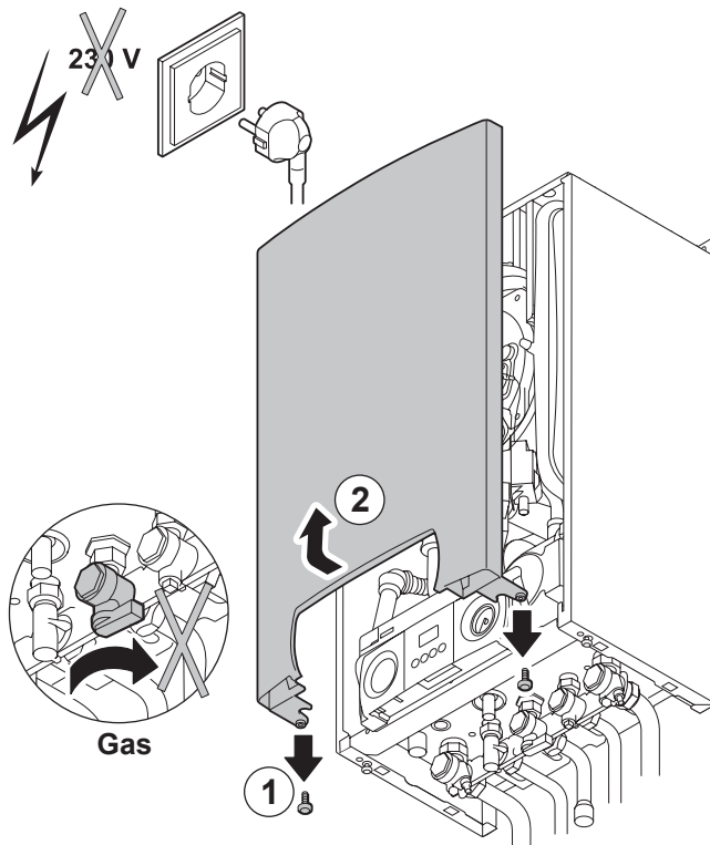
Bild 50 Öffnen des Kessels 111572.LT.DE.W7H.030
