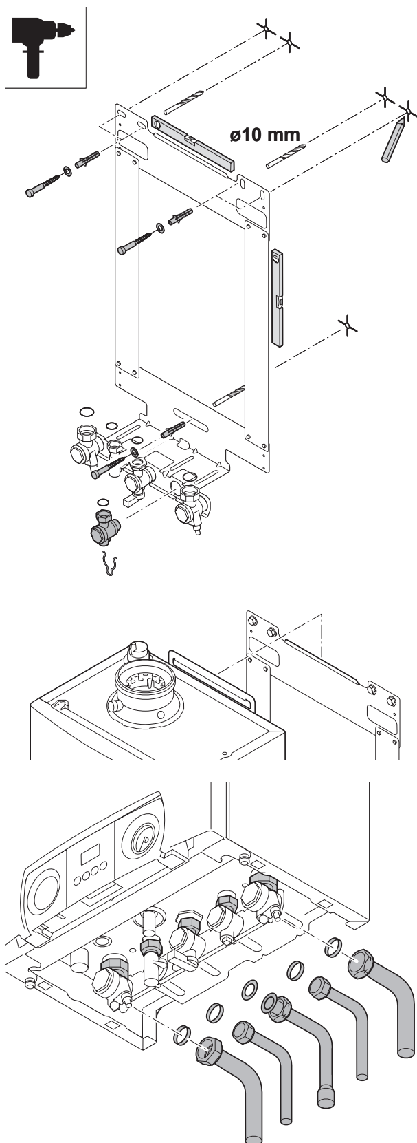
Bild 06 Montage des AvantaPlus
