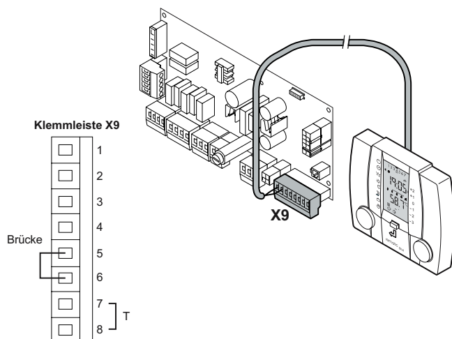
Bild 20 Schaltplan modulierende Steuerung 111572.LT.DE.W7H.009
