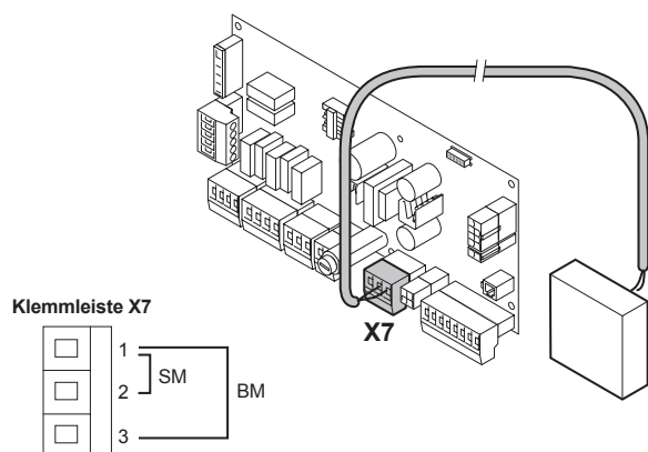
Bild 25 Anschluss Störmeldung 111572.LT.DE.W7H.014
