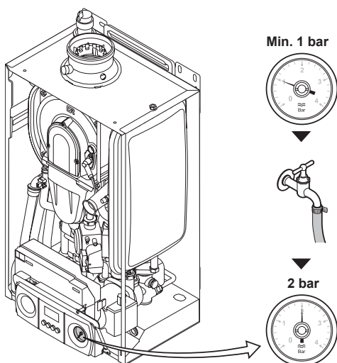
Bild 45 Kontrolle des Wasserdrucks
