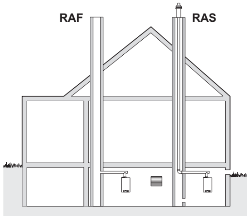
Bild 13 Raumluftabhängiger Betrieb 111572.LT.DE.W7H.004
