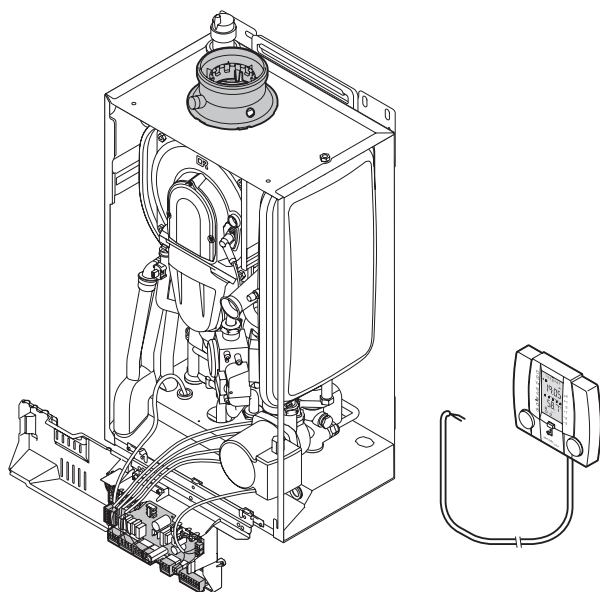
Bild 32 Anschlüsse und Regler prüfen 111572.LT.DE.V7H.018
