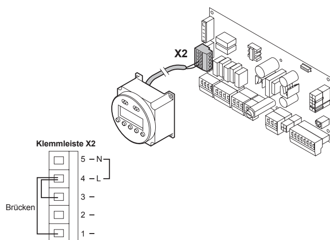
Bild 19 Schaltplan für eine externe 230-V-Zeitschaltuhr 111572.LT.DE.W7H.008
