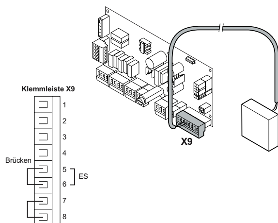
Bild 24 Schalttafel für eine externe Sicherheitseinrichtung
