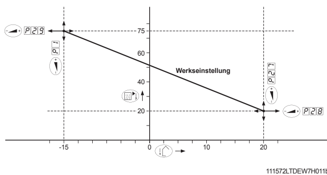
Bild 22 Heizkurve Remeha AvantaPlus 111572.LT.DE.W7H.011
