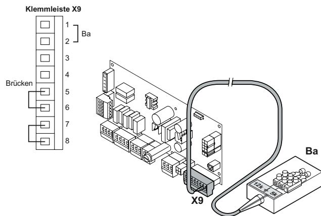
Bild 21 Schaltplan Außentemperatursensor 111572.LT.DE.W7H.010
