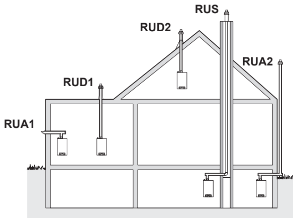
Bild 14 Raumluftunabhängiger Betrieb 111572.LT.DE.W7H.005
