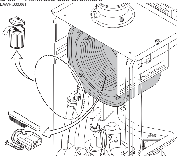
Bild 53 Kontrolle des Brenners
