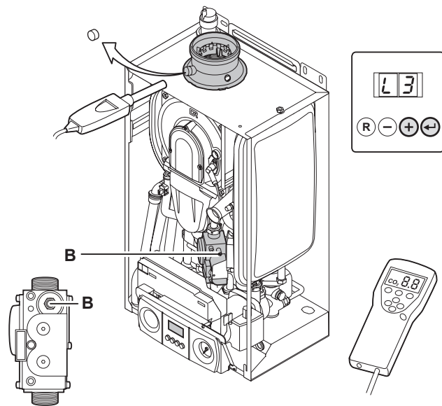
Bild 35 Prüfung der Gas-/Luftverhältnissteuerung – bei Teillast – Gas-/Luftverhältnis Einstellung B am Gasblock
